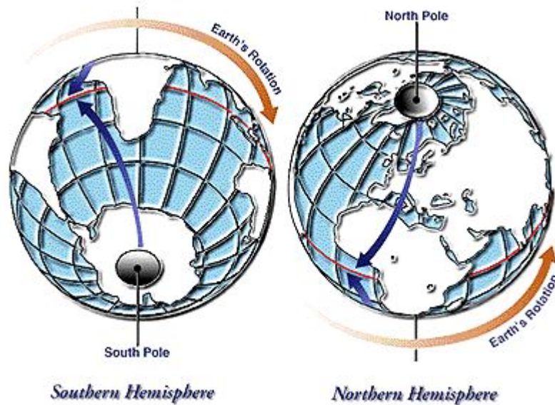
تأثیر نیروی Coriolis در باد
